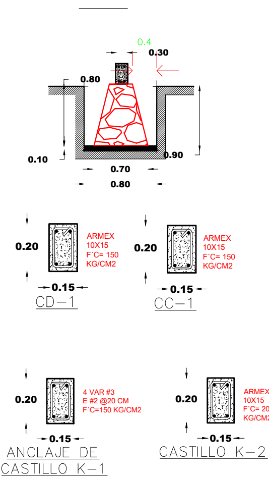
DETALLES CONSTRUCTIVOS
