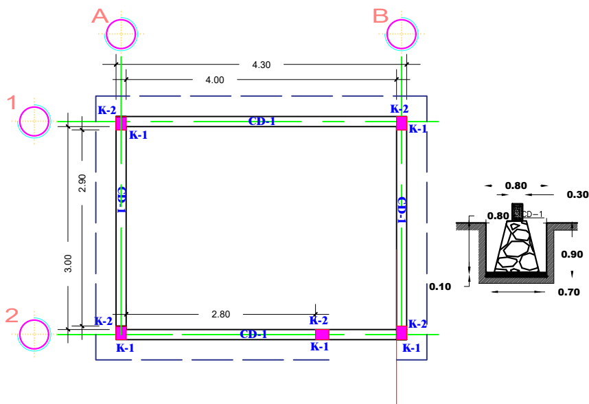
PLANTA DE CIMENTACION
