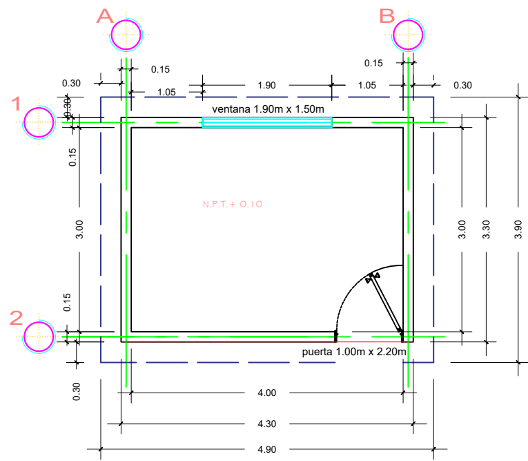
PLANTA ARQUITECTONICO
